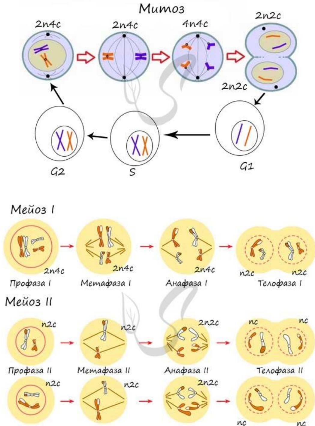
Рис. 4. Сравнение хромосомного цикла при митозе и при мейозе. Указано число хромосом ( n ) и количество ДНК ( c ) на клетку (на одно ядро в телофазе). Кроссинговер происходит в профазе первого деления мейоза 1
